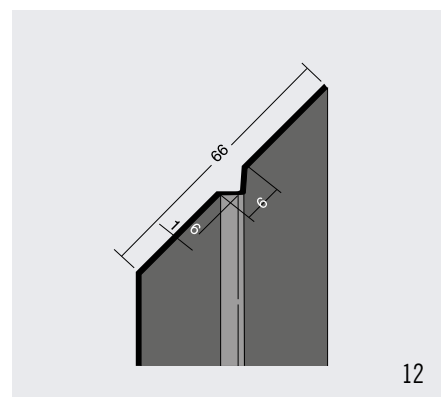
Voegprofiel
